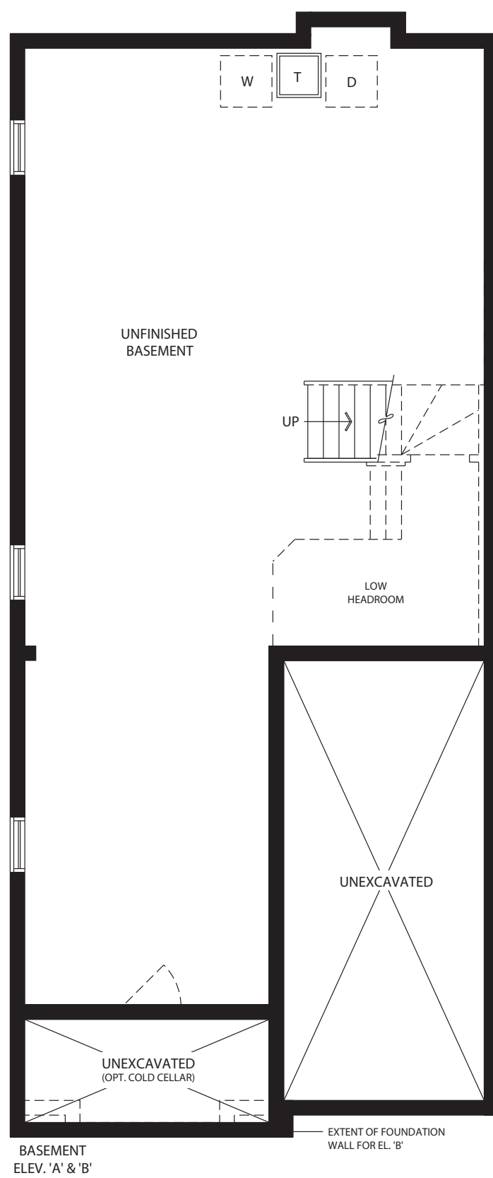
BASEMENT ELEV. 'A' & 'B'
